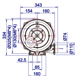
HTB75-032 2-stage
