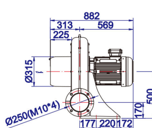
TB150L-10
